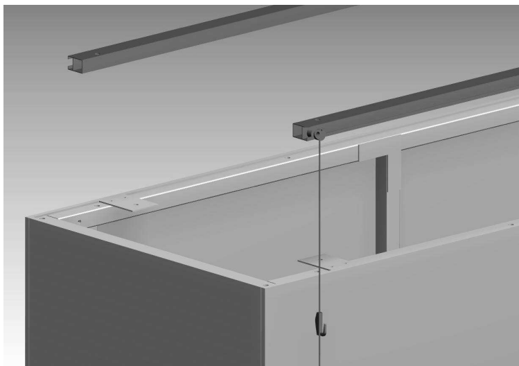
Ilustracja 2. Mocowanie listwy aluminiowej do zawieszania obrazów LM-10
